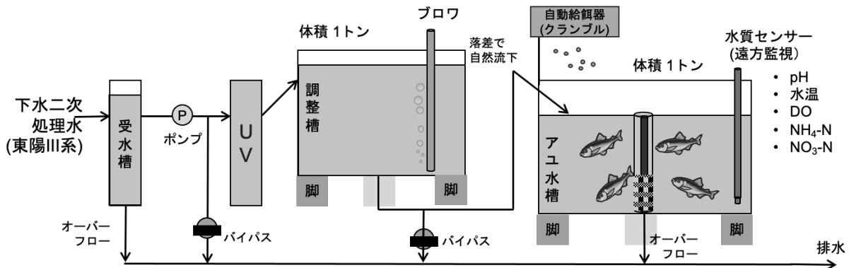
実験施設のフロー図
